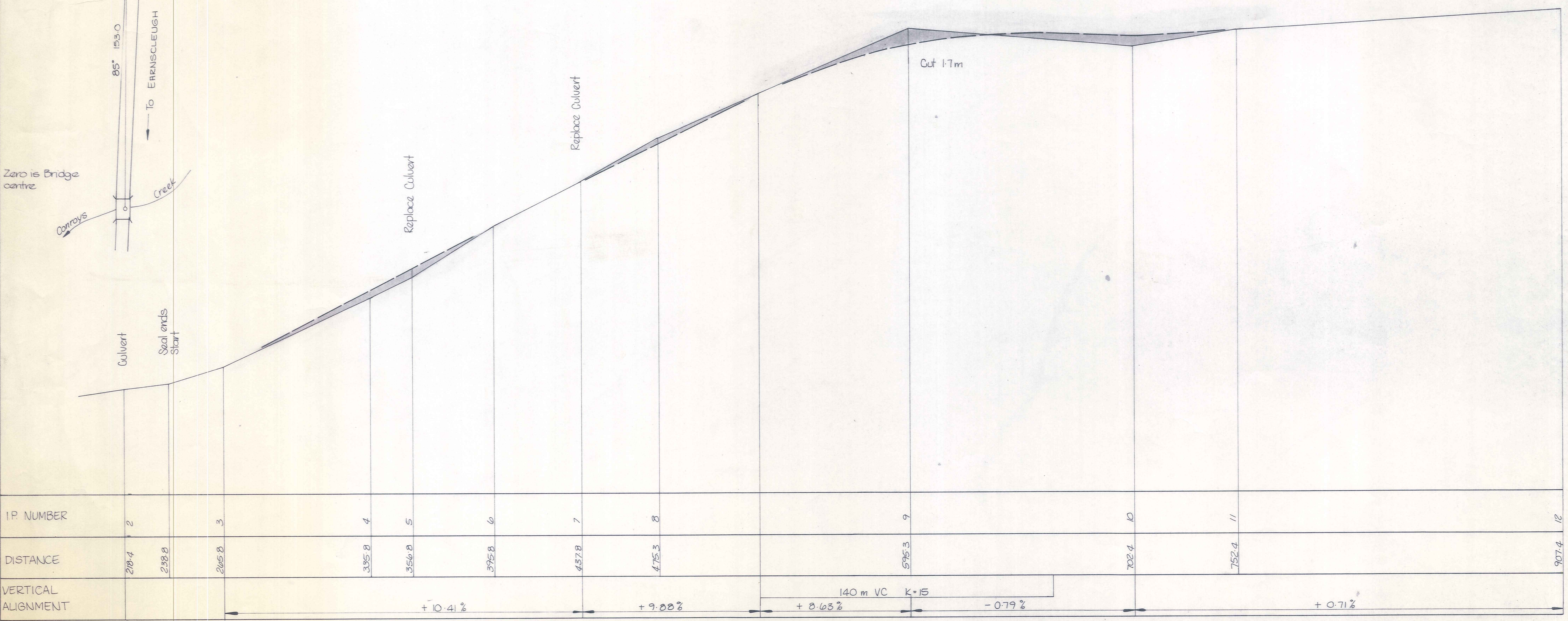
LONGITUDINAL SECTION Horiz: 1:1000 Vert: 1:200
