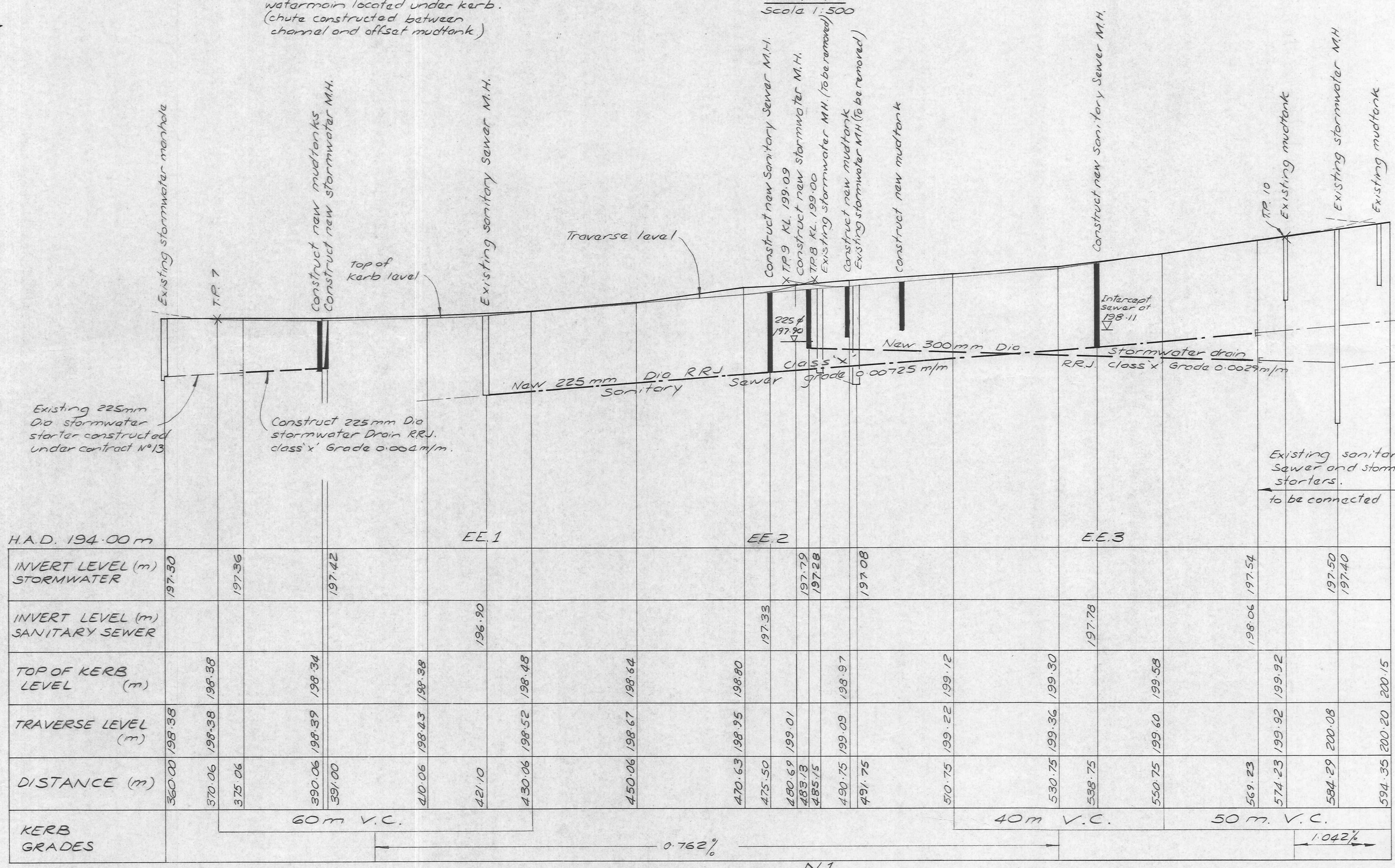
N.1. LONGITUDINAL SECTION Scale: HORIZ 1:500 VERT 1:50
