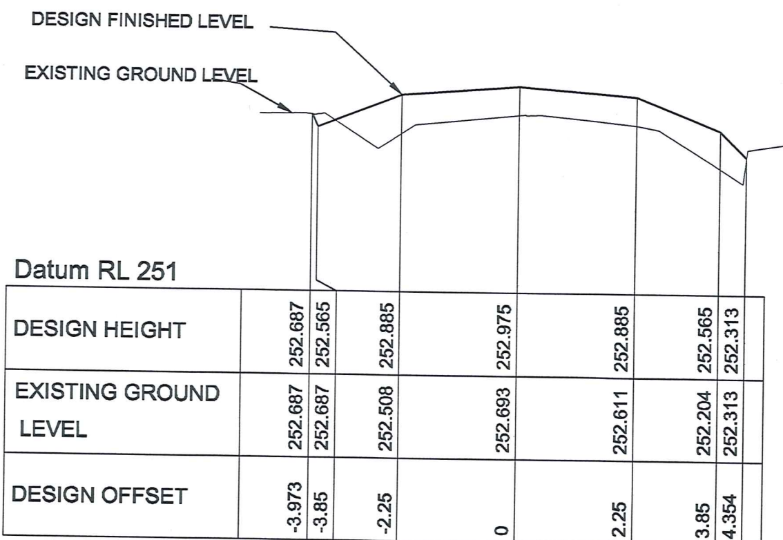
CHAINAGE 350
