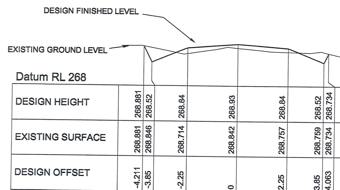
CHAINAGE 200
