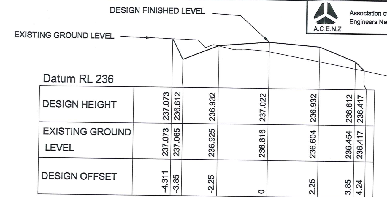
CHAINAGE 790
