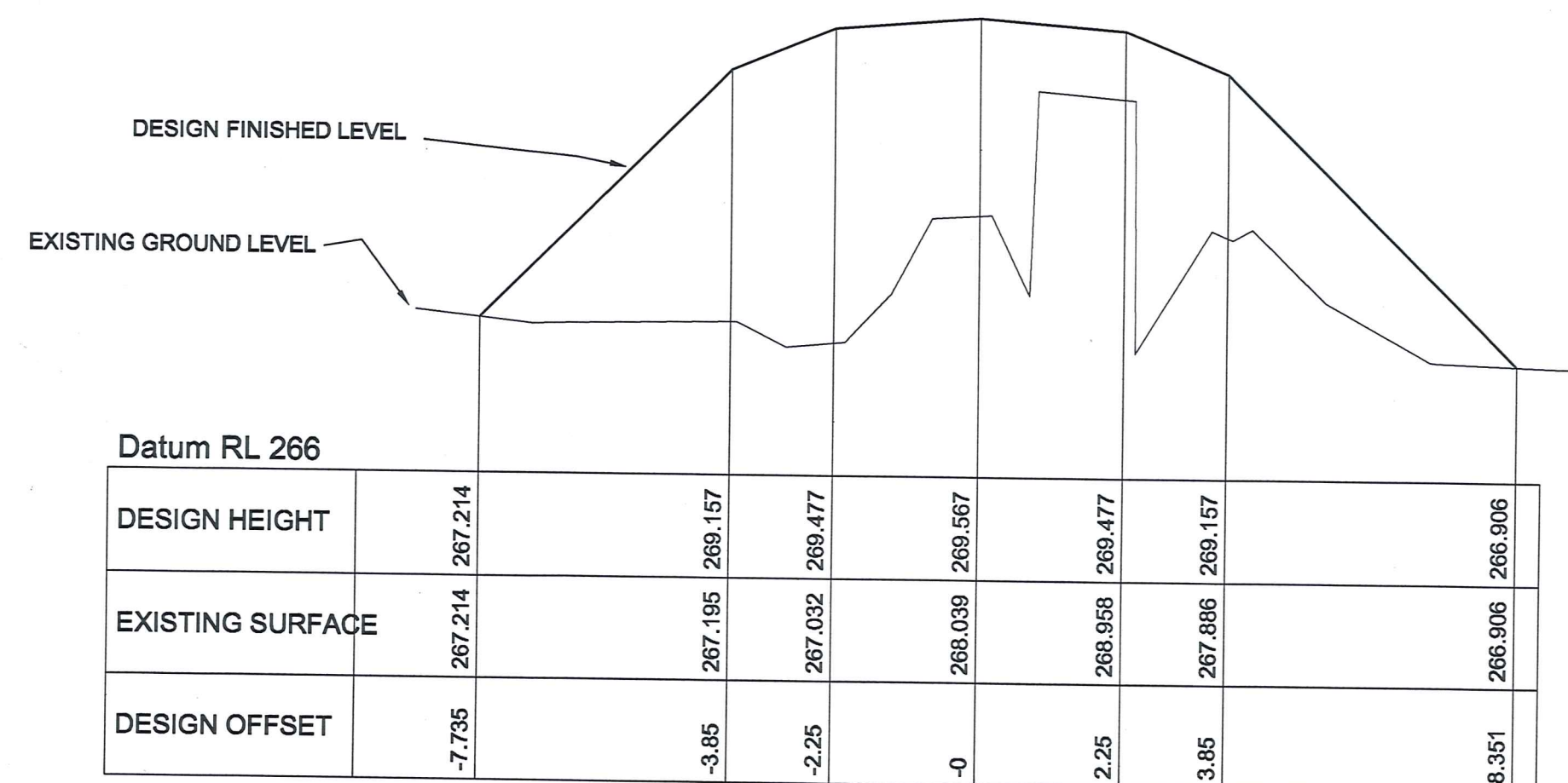
CHAINAGE 100
