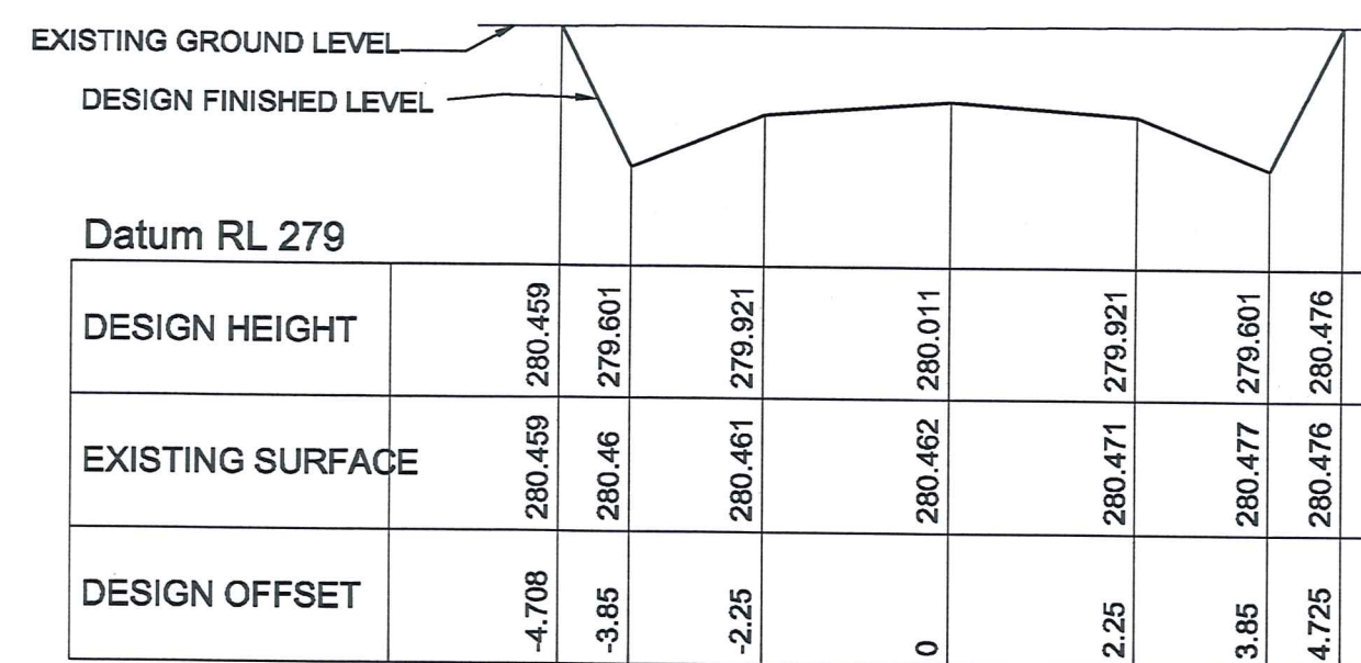
CHAINAGE 550
