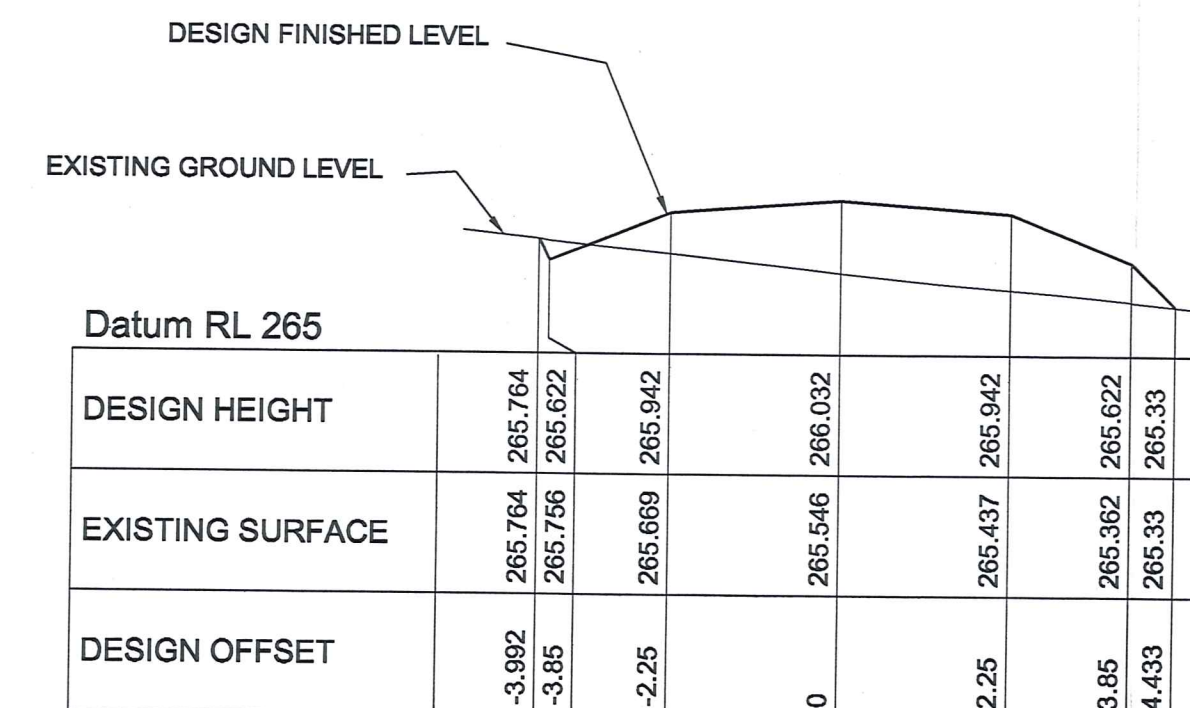
CHAINAGE 350
