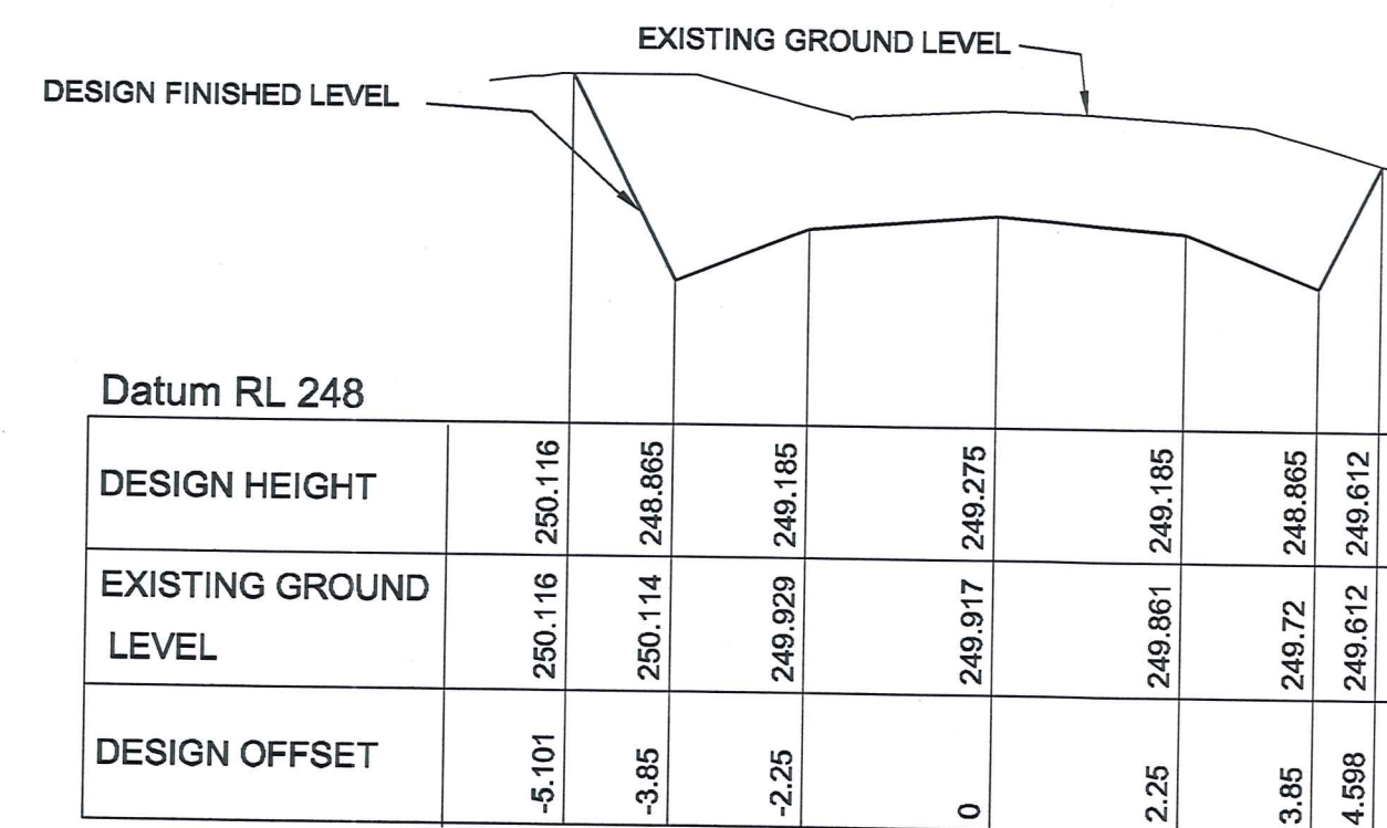
CHAINAGE 500
