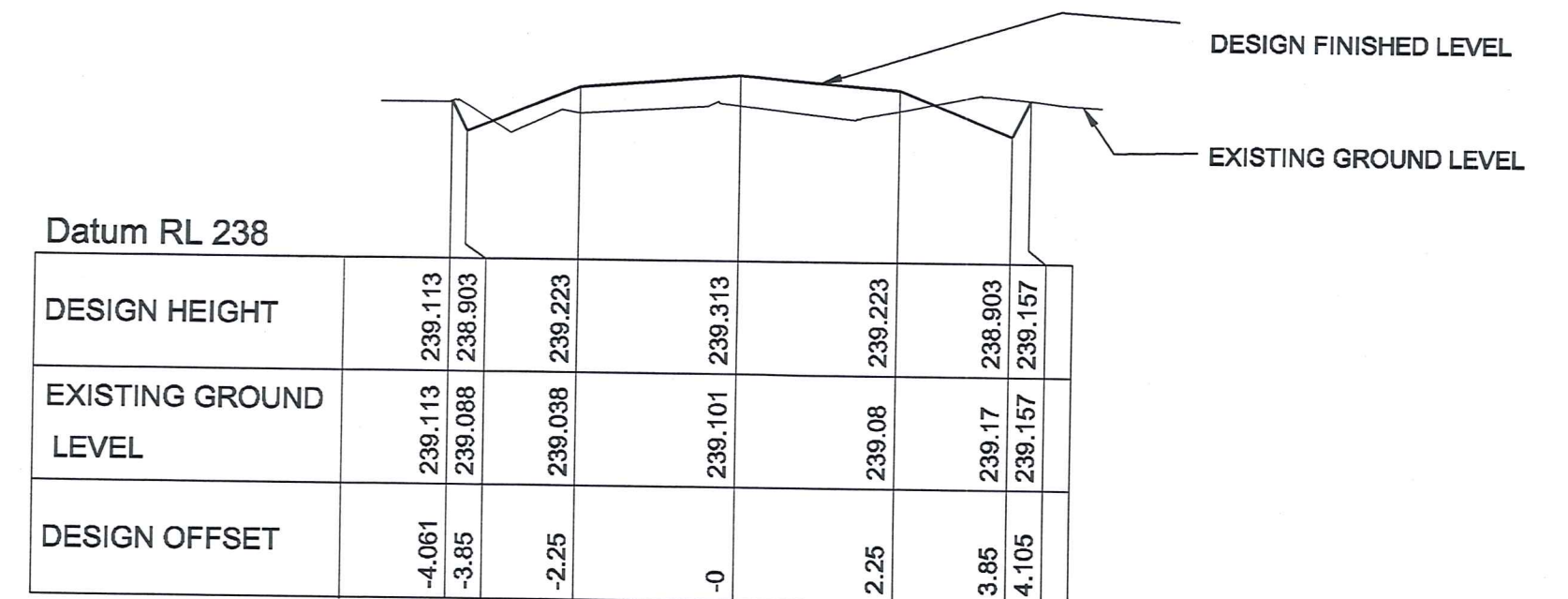
CHAINAGE 650
