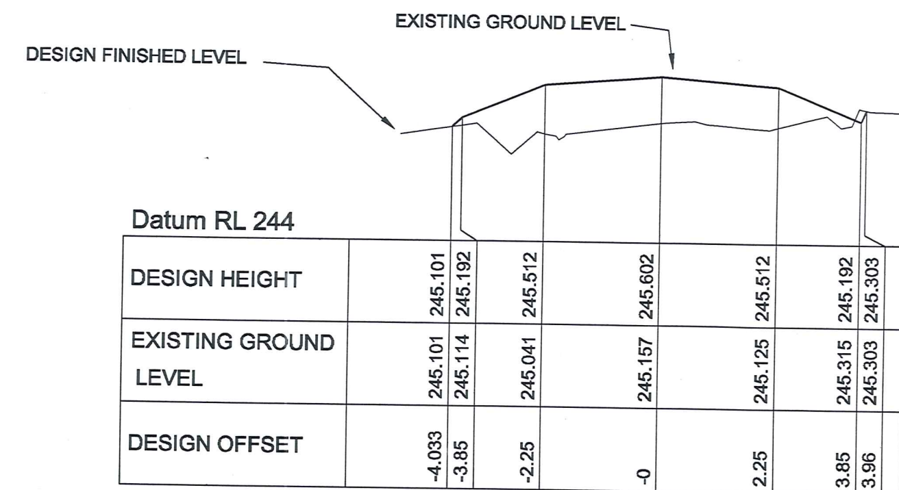
CHAINAGE 550
