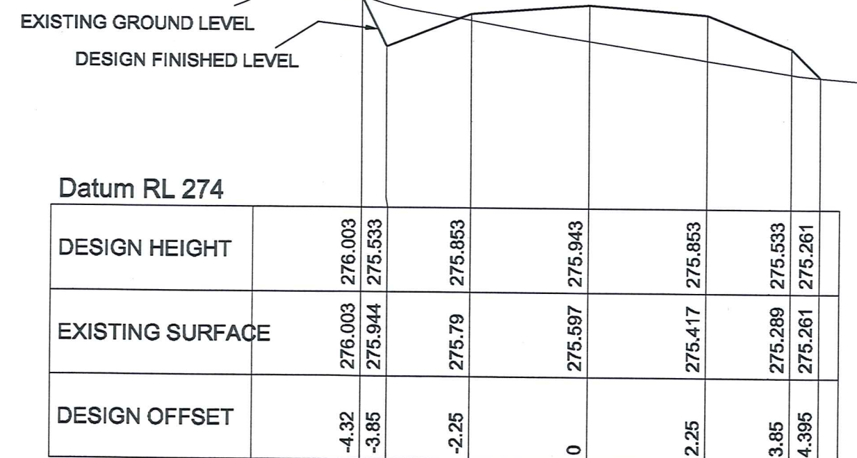
CHAINAGE 650
