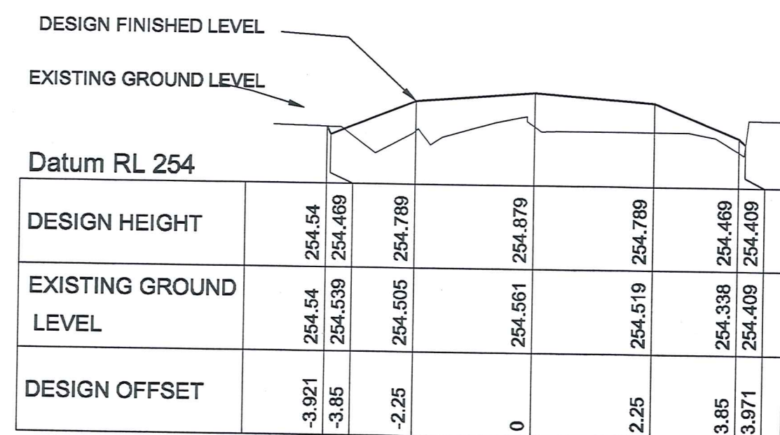
CHAINAGE 300
