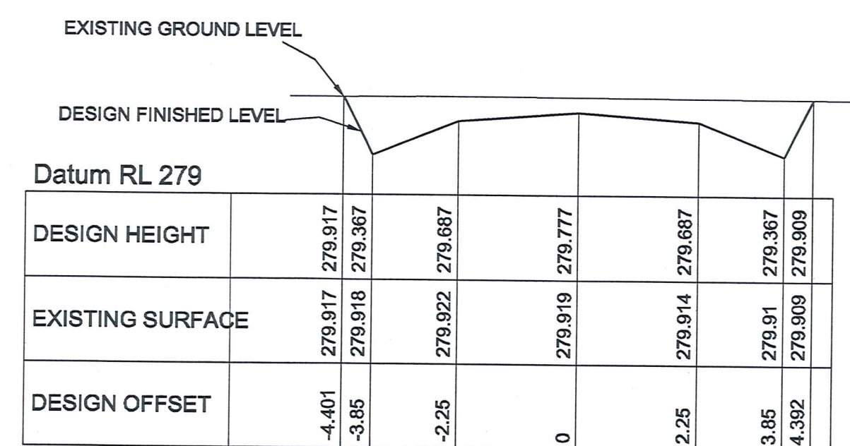
CHAINAGE 600
