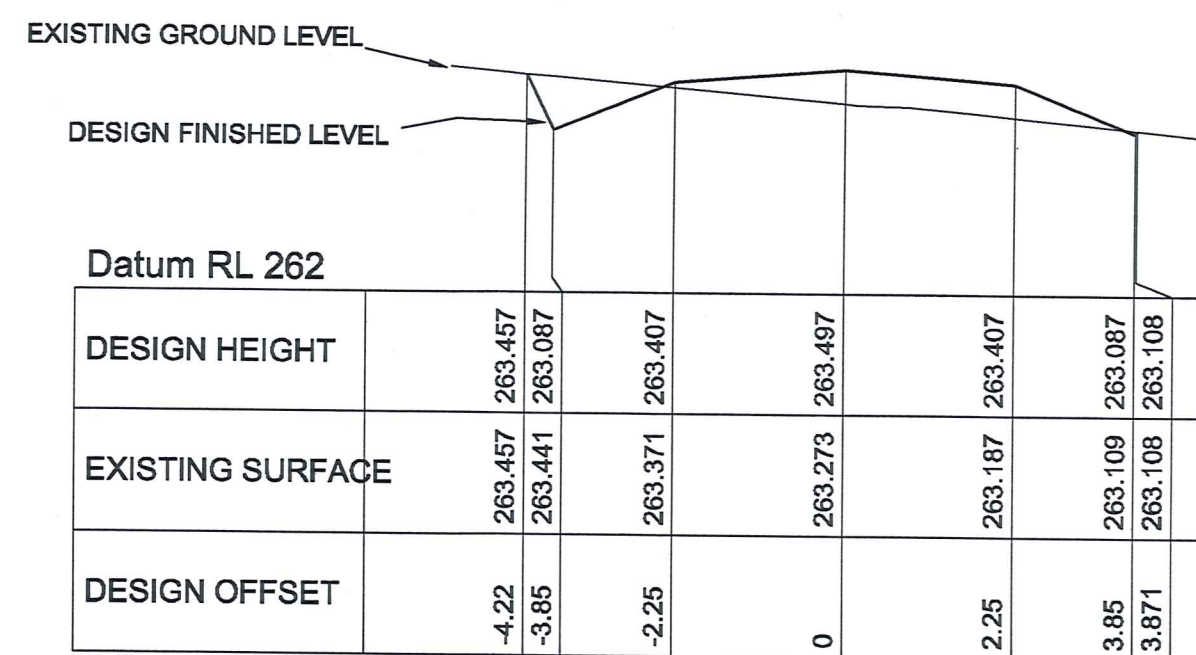
CHAINAGE 400
