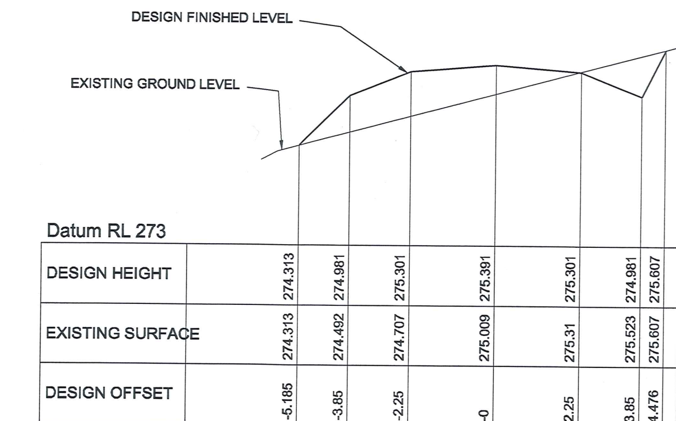
CHAINAGE 750
