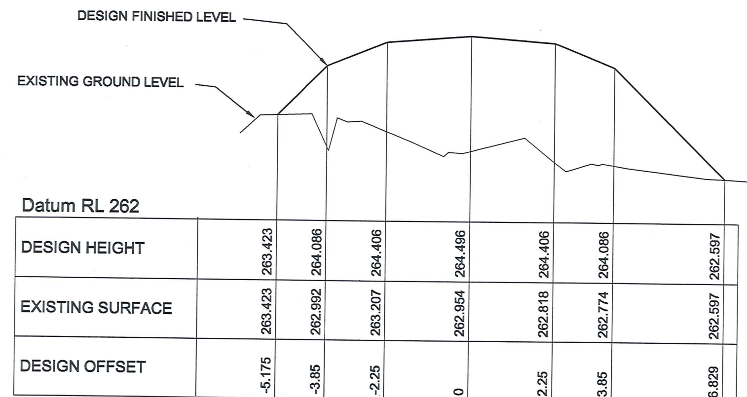
CHAINAGE 250
