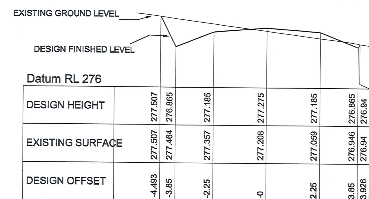
CHAINAGE 700
