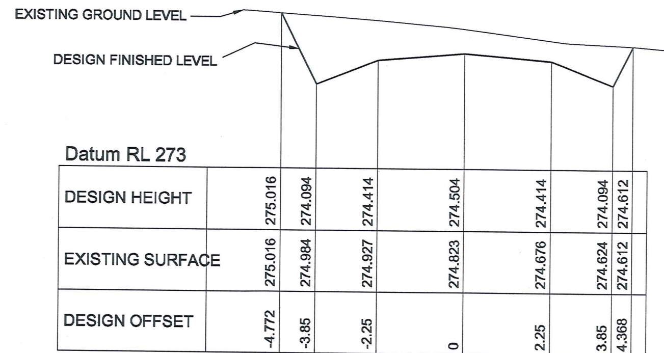
CHAINAGE 500
