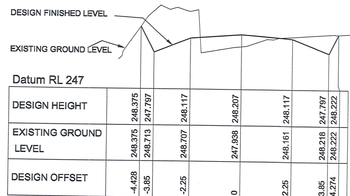
CHAINAGE 400
