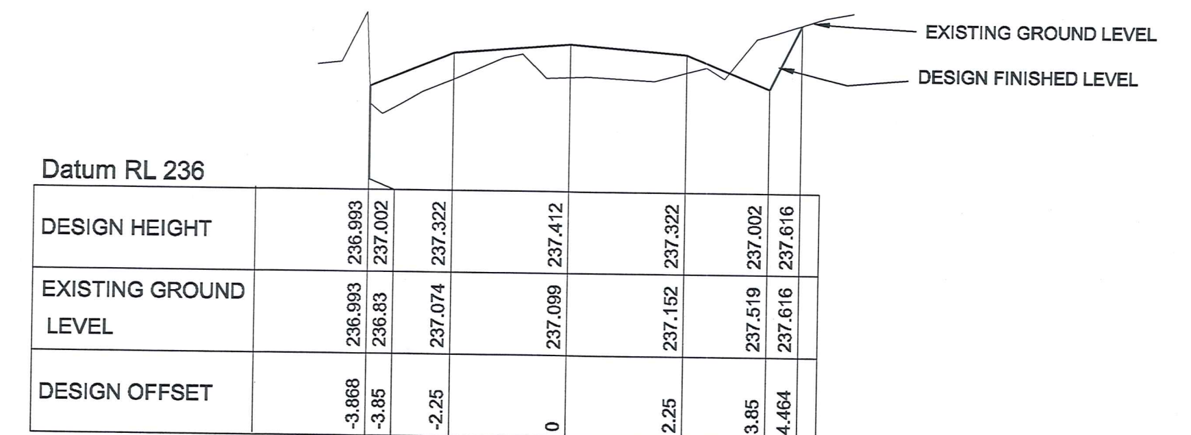
CHAINAGE 700
