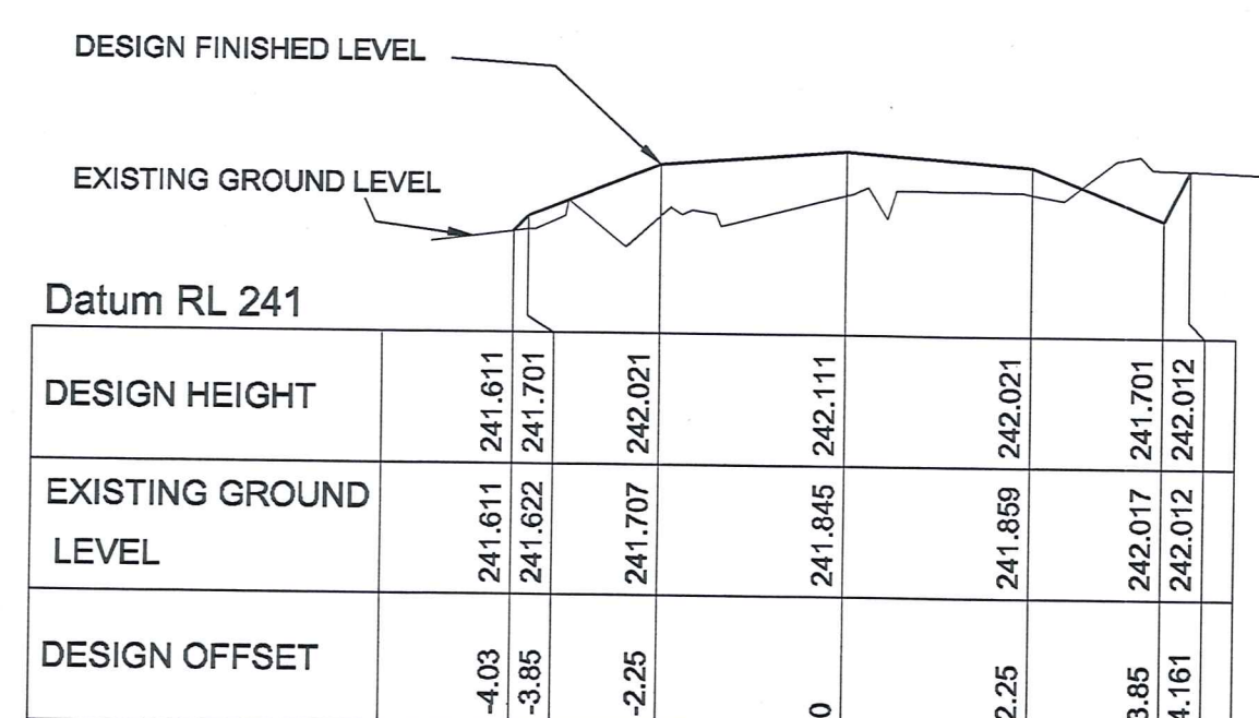
CHAINAGE 600.000
