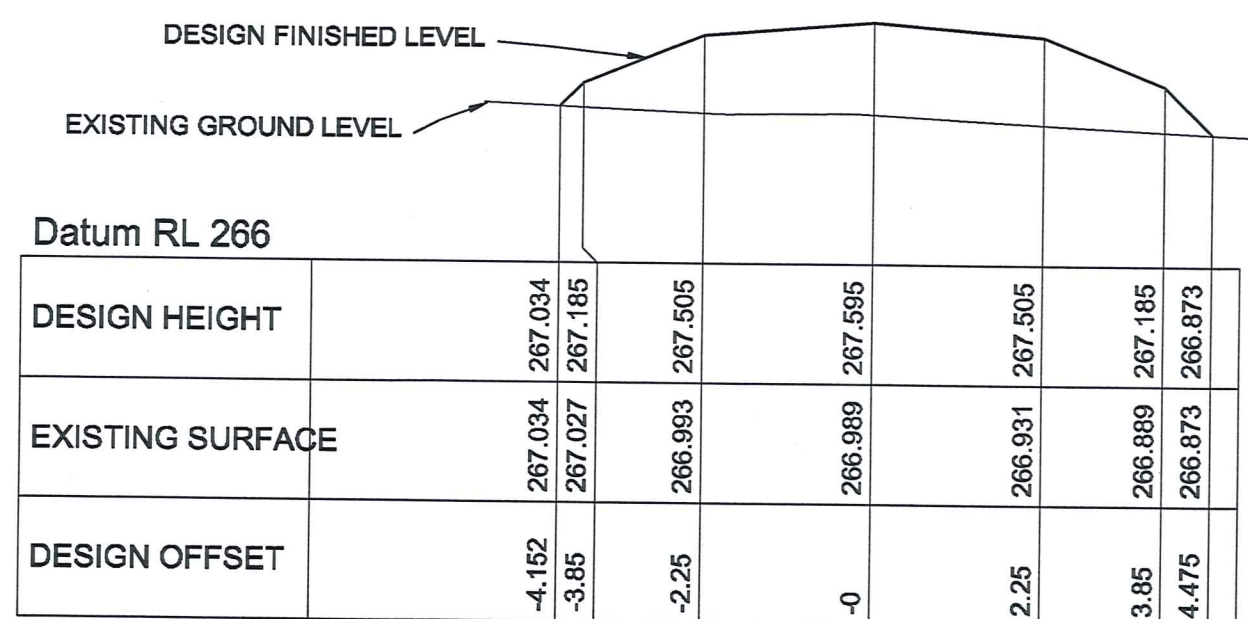
CHAINAGE 450
