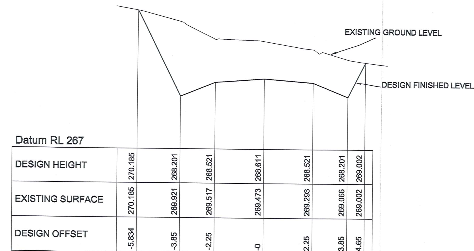
CHAINAGE 300
