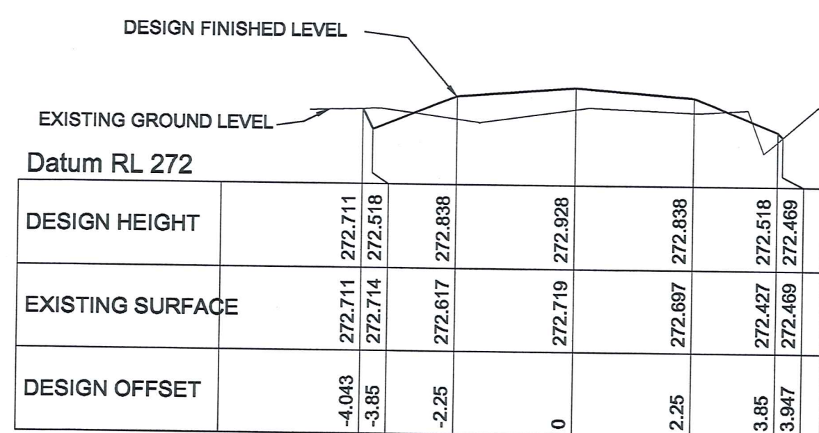
CHAINAGE 50
