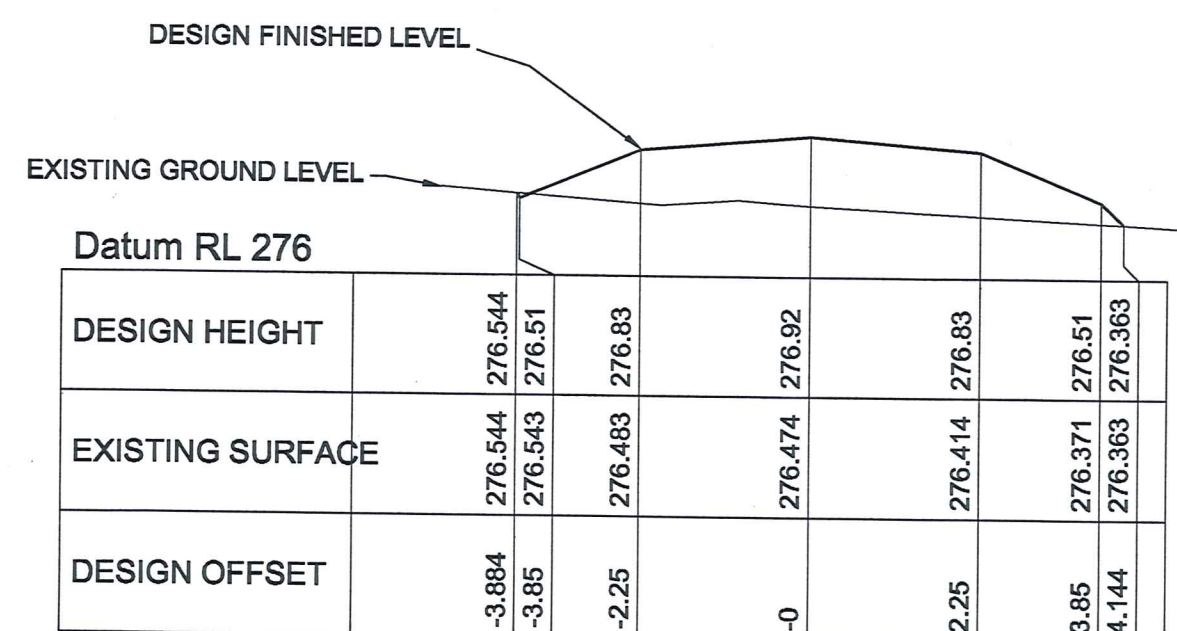
CHAINAGE 0
