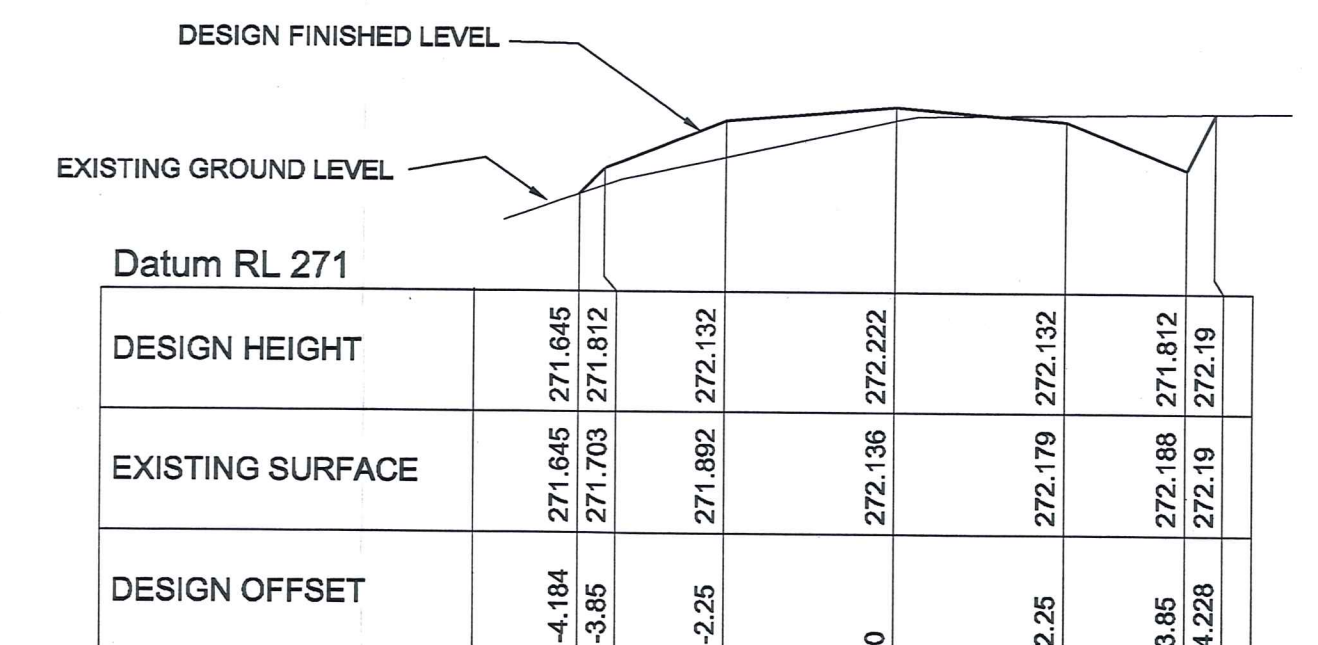
CHAINAGE 800
