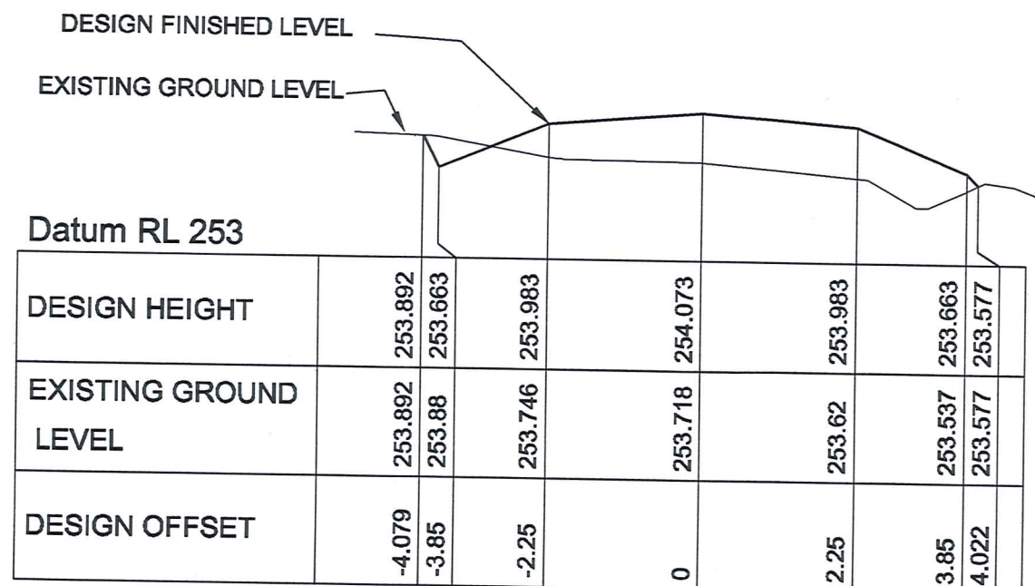
CHAINAGE 150
