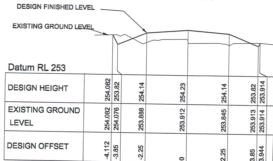
CHAINAGE 100
