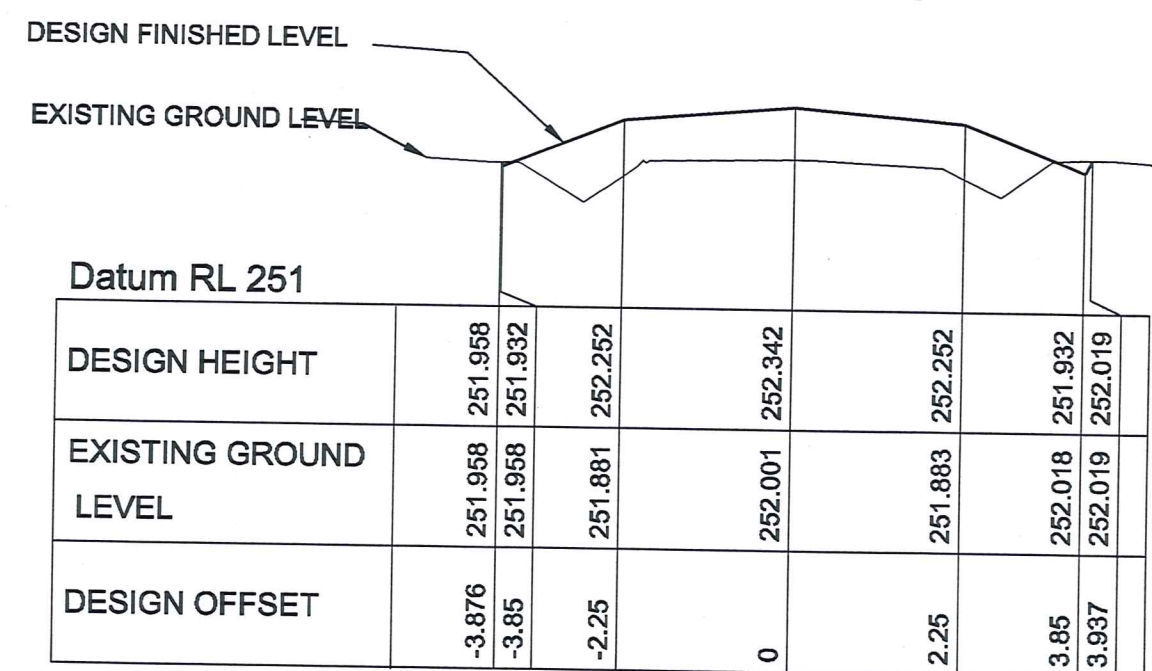
CHAINAGE 50
