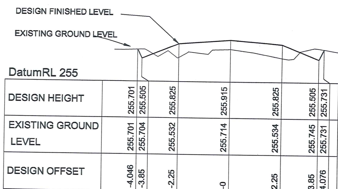
CHAINAGE 250
