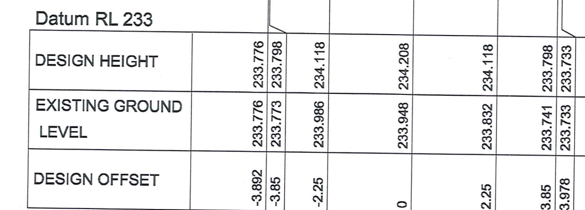
CHAINAGE 750
