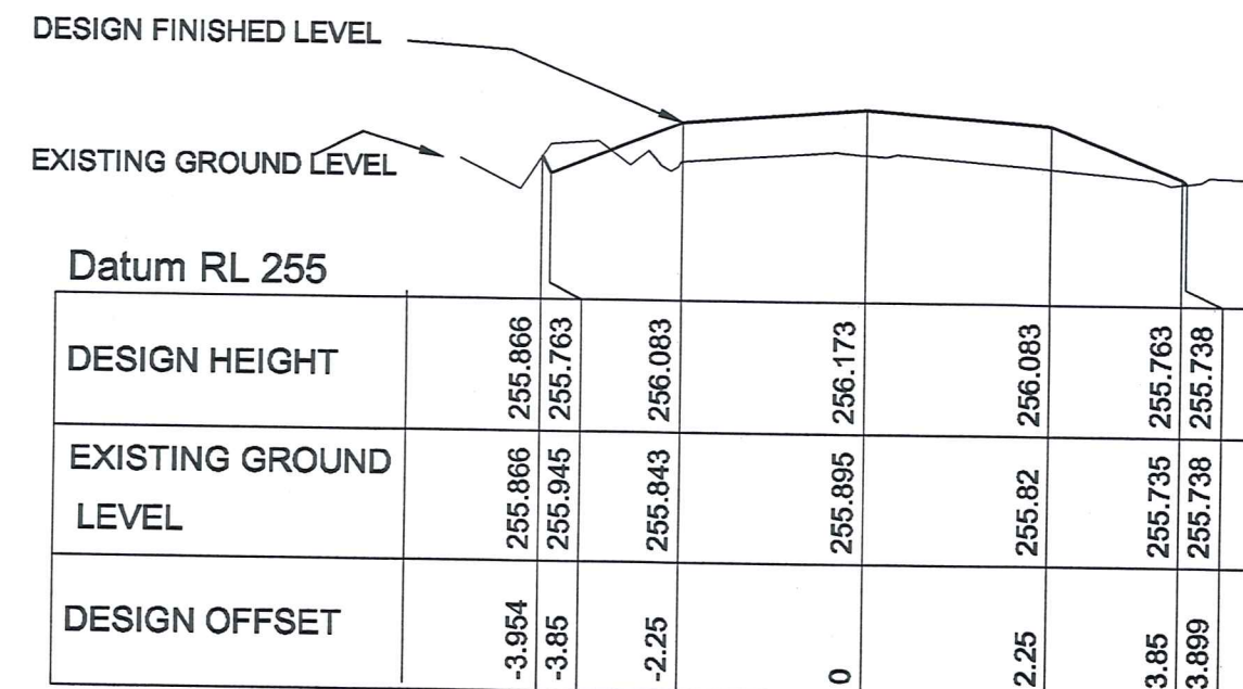
CHAINAGE 200
