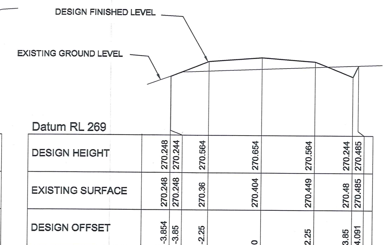
CHAINAGE 820.906
