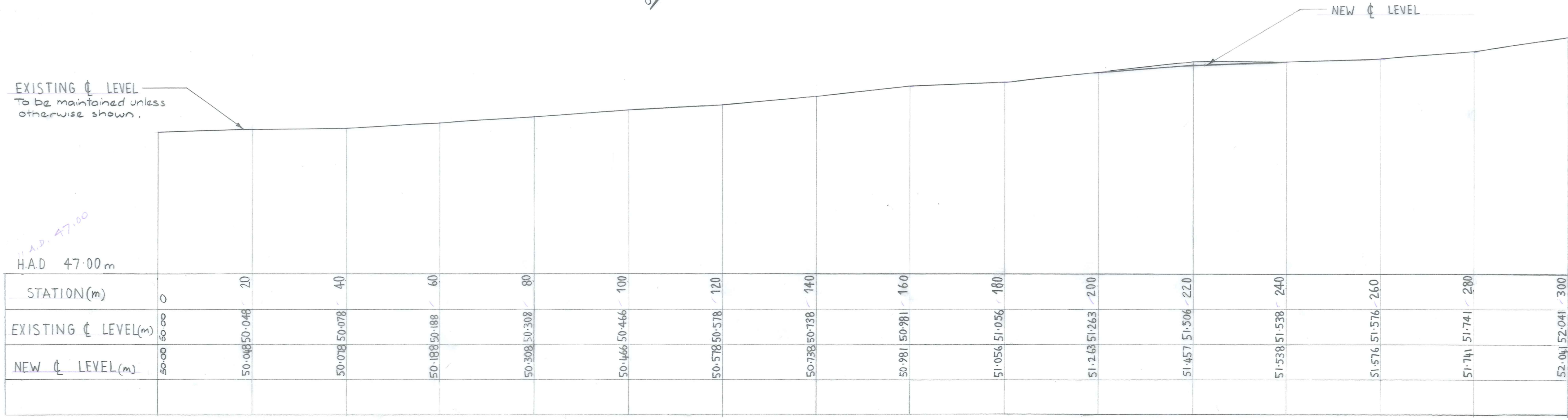
LONGITUDINAL SECTION Scales: Horz. 1:500 Vert. 1:50
