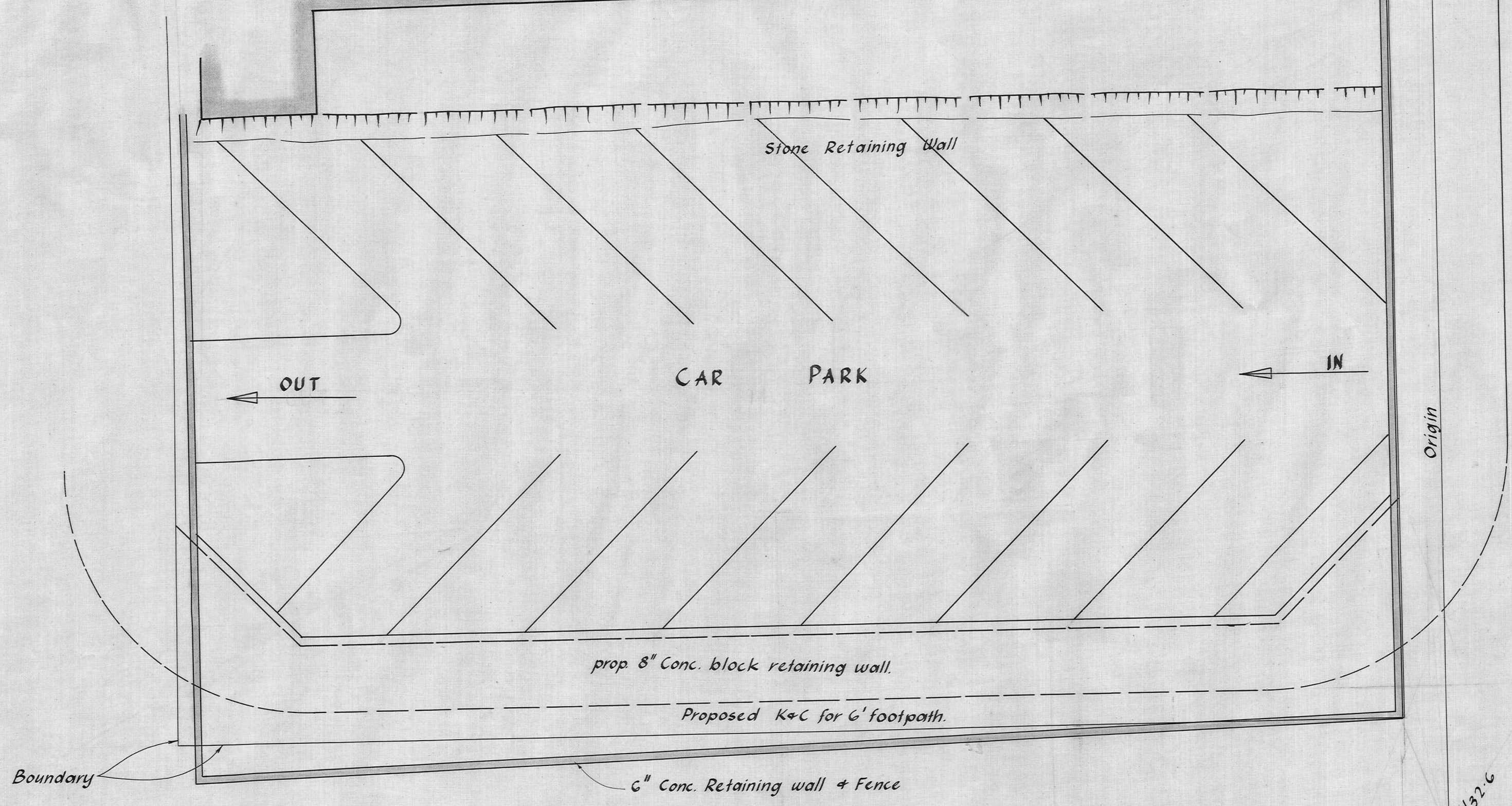
-DETAIL A- Scale: 1/8 inch = 1 foot.
