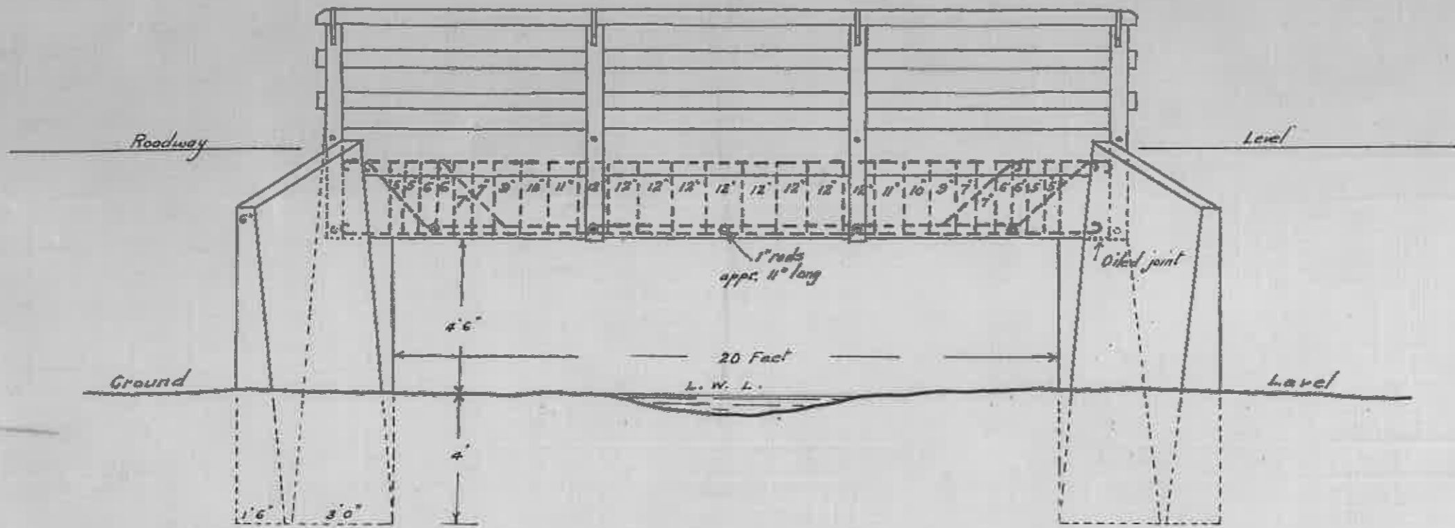
Elevation
